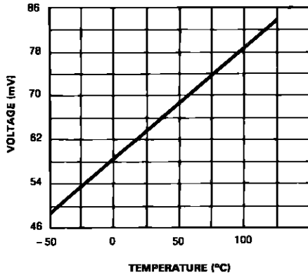
TURN-ON VOLTAGE
