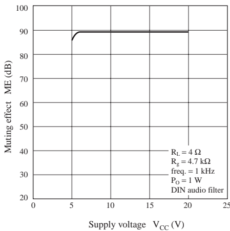
ME — V_{CC}
