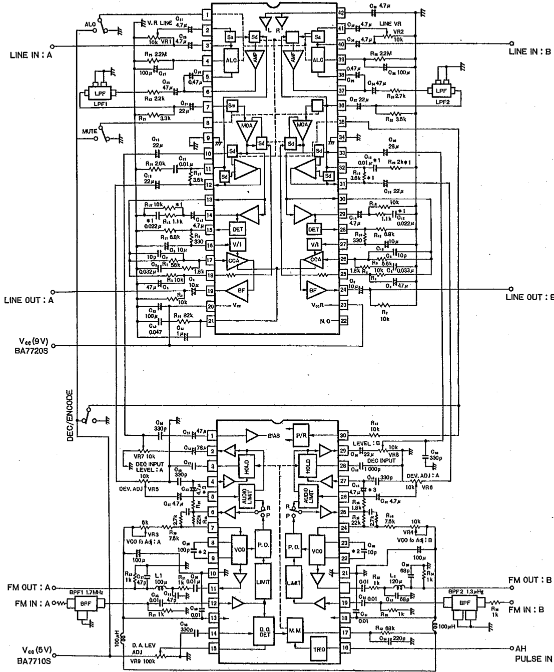
VR : RVQ0707 タイプ(ムラタ) *1 許容差 R : ±2% C : ±5% BPF1 : LJ25BP1.7M01-32(ムラタ) *2 温度特性 ±0ppm 許容差 ±5% BPF2 : LJ25BP1.3M02-32(ムラタ) *3 無極性コンデンサ LPF1, 2 : 75B-122-074(スミダ) 単位 R : Ω L : R0855 タイプ(スミダ) Fig.1
