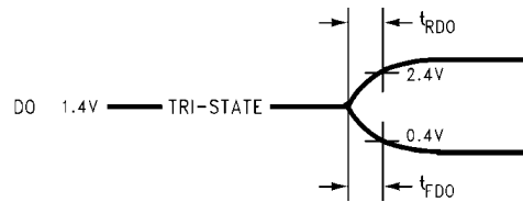
DO "TRI-STATE" Falling and Rising Edge
