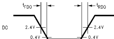
DO Falling and Rising Edge
