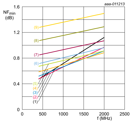
V CE = 8 V; T amb = 25 °C; Γ S = Γ opt . (1) I C = 1 mA (2) I C = 2 mA (3) I C = 3 mA (4) I C = 5 mA (5) I C = 8 mA (6) I C = 10 mA (7) I C = 15 mA (8) I C = 25 mA (9) I C = 35 mA
