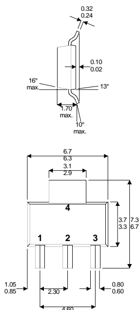
SOT-223
