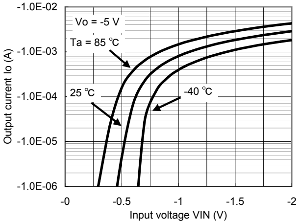
Io - VIN
