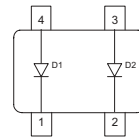
BAT68-07W
