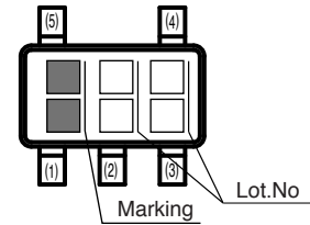
BD45XXXG/BD46XXXG : SSOP5(SMP5C2)
