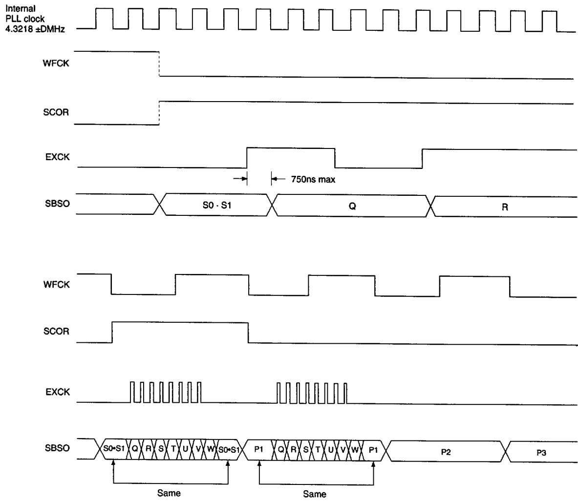
Subcode P.Q.R.S.T.U.V.W Read Timing
