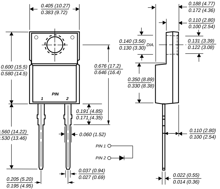
ITO-220AC (FESF8JT)
