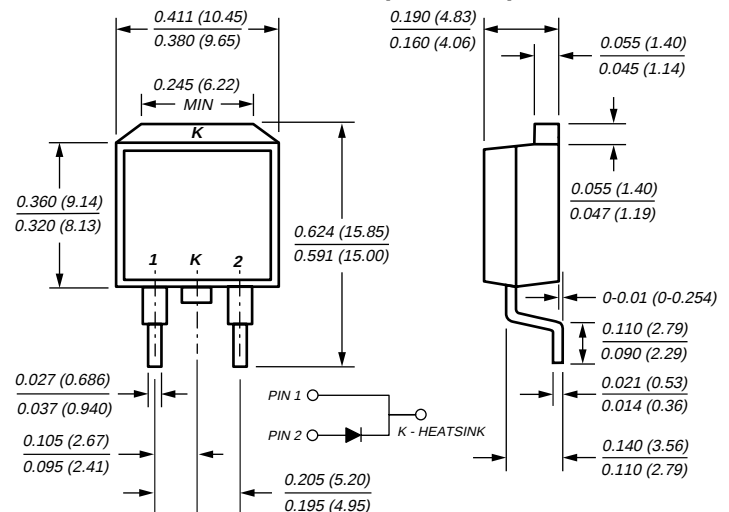
TO-263AB (FESB8JT)
