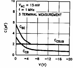
C BE , C CSUB , C CB vs Voltage
