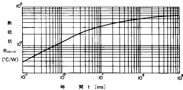
熱抵抗 R_{th(j-c)} (°C/W) 時間 t (ms) 過渡熱抵抗(ダイオード)特性 Transient Thermal Resistance (Diode)
