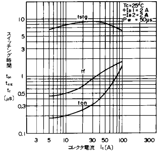
スイッチング時間 t_{stg} t_f t_{on} t_r コレクタ電流 I_c (A) スイッチング時間—コレクタ電流特性 Switching Time
