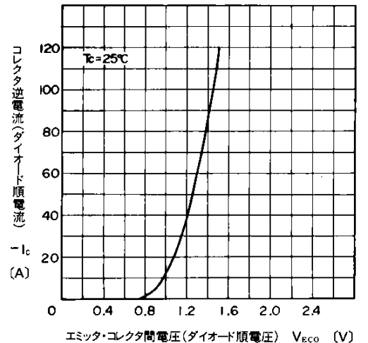
コレクタ逆電流(ダイオード順電流) -I_c (A) エミッタ・コレクタ間電圧(ダイオード順電圧) V_{ceo} (V) 高速フリーホイリングダイオード順特性 Forward Voltage of Free Wheeling Diode
