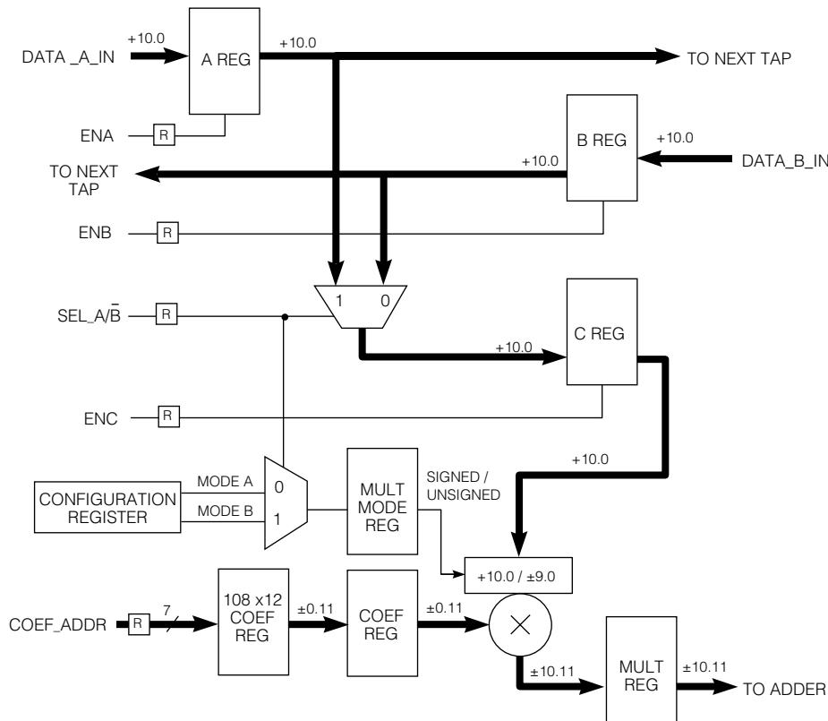
Fig. 4 Tap Cell (1-12)
