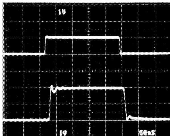
Vertical Scale: V_{IN} = 1\text{V/Div.} , V_{OUT} = 1\text{V/Div.} Horizontal Scale: 50ns/Div.
