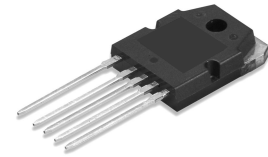
1.DRAIN 2. GND 3. V CC 4. FB 5. S/S
