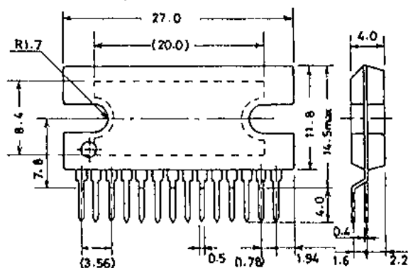
Case Outline 3113-S14HZ IC (unit : mm)
