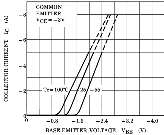
I_C - V_{BE}
