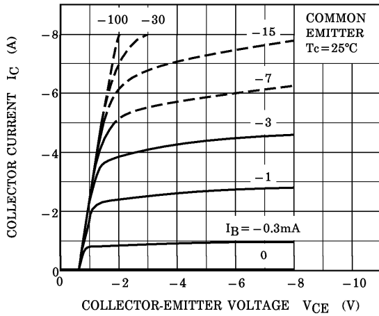
I_C - V_{CE}
