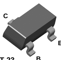
SOT-23 Mark: 1P
