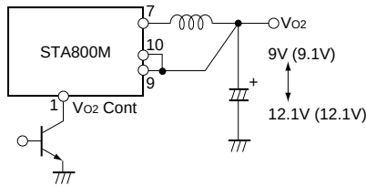
Vo 2 output voltage
