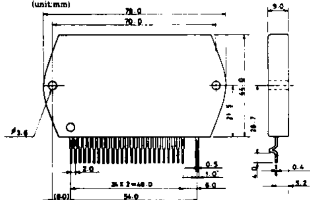
外形図 4091 (unit:mm)
