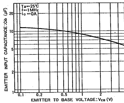
Fig.12 エミッタ入力容量—エミッタ・ベース電圧特性
