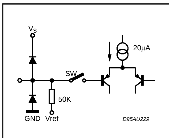
PIN: REARIN
