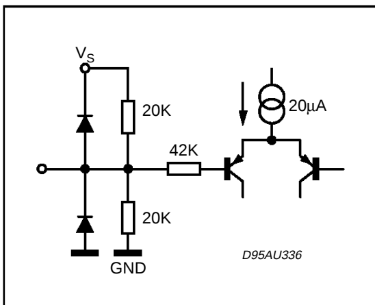
PIN: CREF
