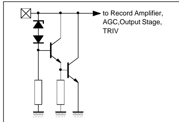
Pin : VCC1
