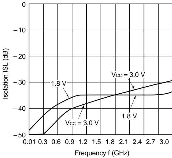
ISL - f
