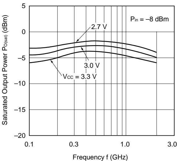
P_{O(sat)} - f
