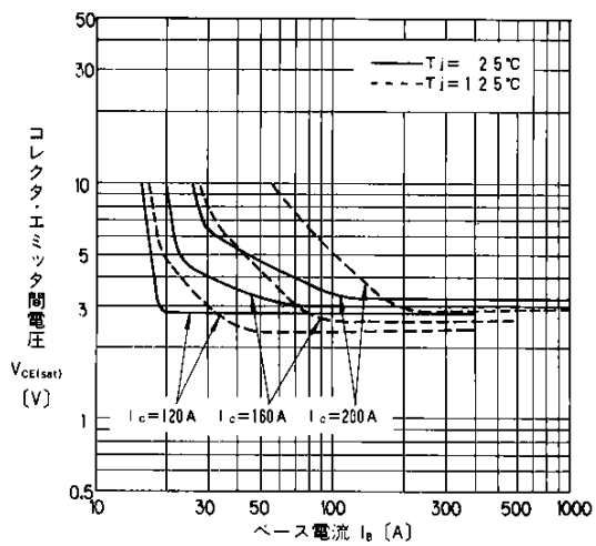
出力特性
