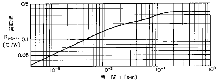
過渡熱抵抗(ダイオード)特性 Transient Thermal Resistance (Diode)
