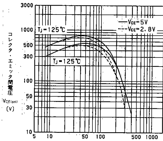
出力特性 Collector Output Characteristics
