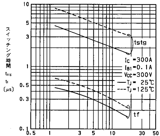
ベース電流 -I_{b2} (A) スイッチング時間-ベース電流特性 Switching Time
