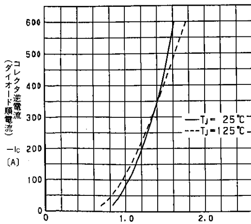
エミッタ-コレクタ間電圧 V_{ec0} (V) (ダイオード順電圧) 高速フリーホイーリングダイオード順電圧特性 Forward Voltage of Free Wheeling Diode
