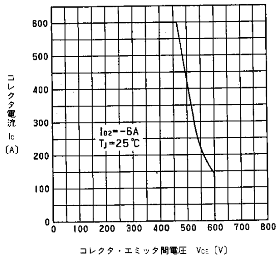
安全動作領域(逆バイアス) Reverse Bias Safe Operating Area
