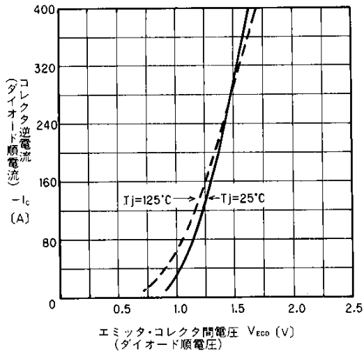
エミッタ・コレクタ間電圧 V_{Eco} (V) (ダイオード順電圧) 高速フリーホイーリングダイオード順電圧 Forward Voltage of Free Wheeling Diode
