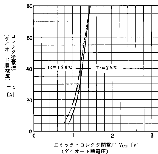
高速フリーホイリングダイオード順電圧
