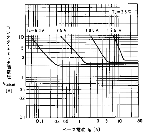
出力特性
