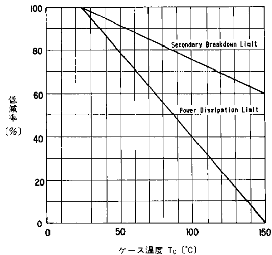
ASO低減特性
