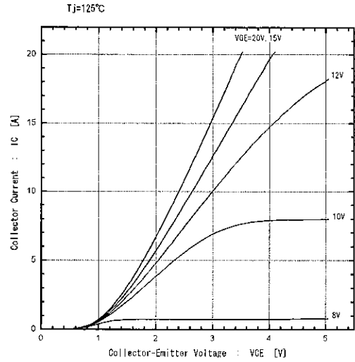
コレクタ電流—コレクタ・エミッタ間電圧特性 Collector current vs. Collector-Emittor voltage
