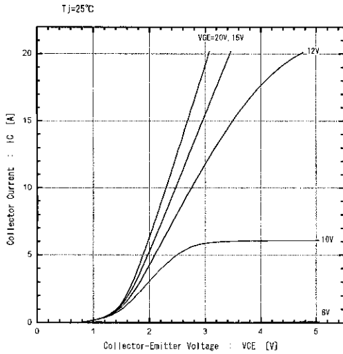
コレクタ電流—コレクタ・エミッタ間電圧特性 Collector current vs. Collector-Emittor voltage
