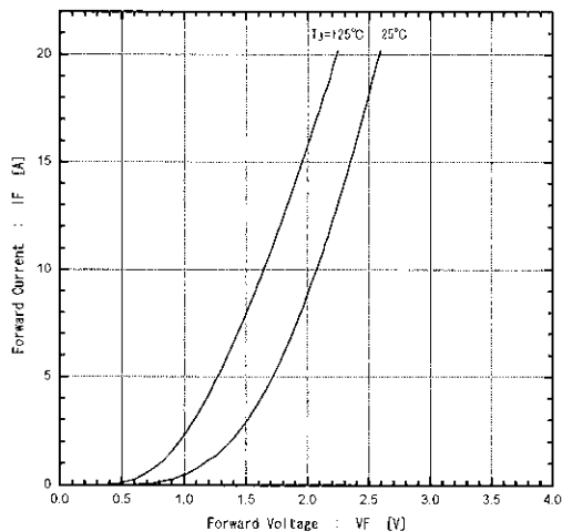
順電流—順電圧特性
