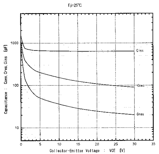
入力・出力・帰還容量—コレクタ・エミッタ間電圧特性 Capacitance vs. Collector-Emmitter voltage
