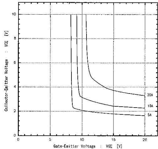
コレクタ・エミッターゲート・エミッタ間電圧特性 Collector-Emittor vs. Gate-Emittor voltage
