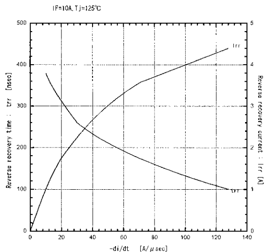
逆回復特性—di/dt
