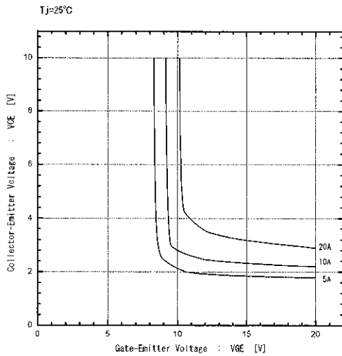
コレクタ・エミッターゲート・エミッタ間電圧特性 Collector-Emittor vs. Gate-Emittor voltage
