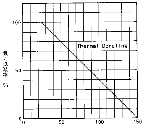
電力低減特性 P_c Derating
