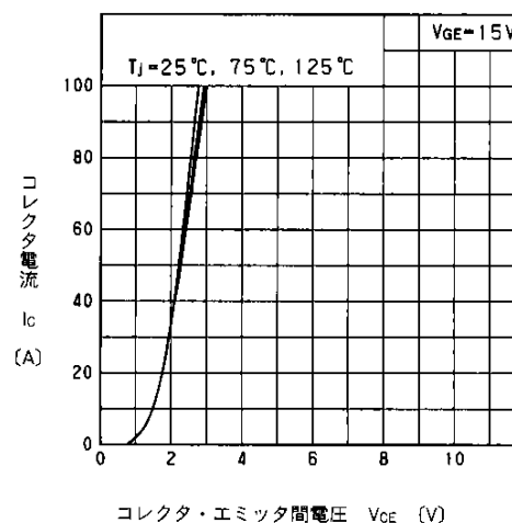
飽和電圧-コレクタ電流特性(標準値)
