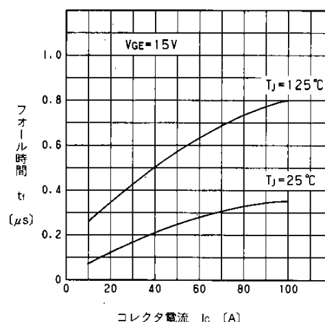
t_f -コレクタ電流特性(標準値)
