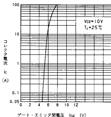
伝達特性(標準値)
