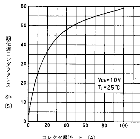
順伝達コンダクタンス-コレクタ電流特性(標準値)
