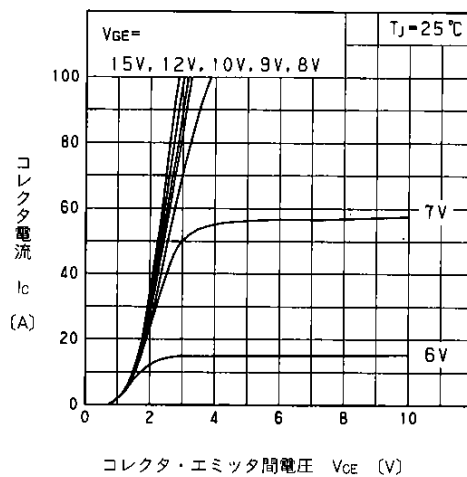
出力特性(標準値)
