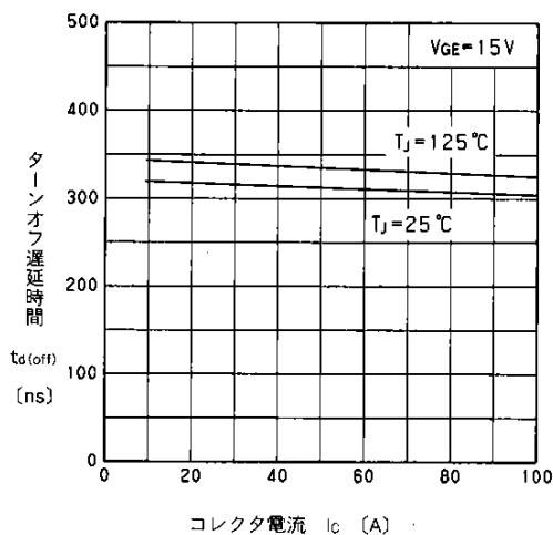
t_{d(off)} -コレクタ電流特性(標準値)
