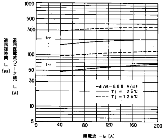
T_{rr} , t_{rr} - I_c 特性 T_{rr} , t_{rr} - I_c
