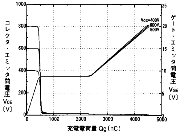
ダイナミック入力特性 ( T_j=25^\circ\text{C} ) Dynamic input characteristic
