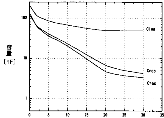
容量-コレクタ・エミッタ間電圧特性 (T J =25°C) Capacitance vs. Collector-Emitter voltage
