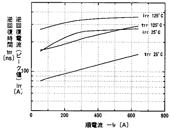
T_{rr} , I_{rr} - I_F 特性 T_{rr} , I_{rr} - I_F
