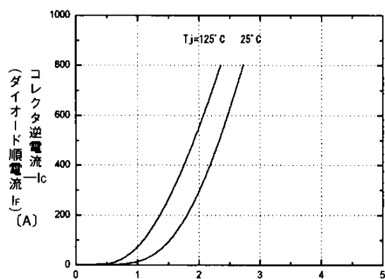
エミッタ・コレクタ間電圧 V_{ce} (V)
