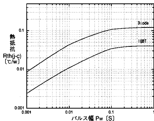
過渡熱抵抗特性 Transient thermal resistance
