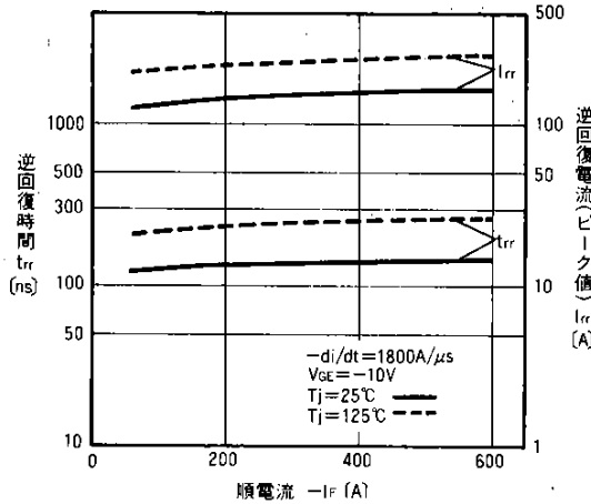
T_{rr} , I_{rr} - I_f 特性 T_{rr} , I_{rr} - I_f
