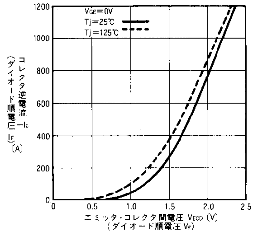
高速フリーホイールダイオード順電圧特性 Forward Voltage of Free Wheeling Diode
