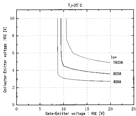
コレクタ・エミッタ間電圧—ゲート・エミッタ間電圧特性 Collector-Emittor voltage vs. Gate-Emittor voltage (Tj=25°C)
