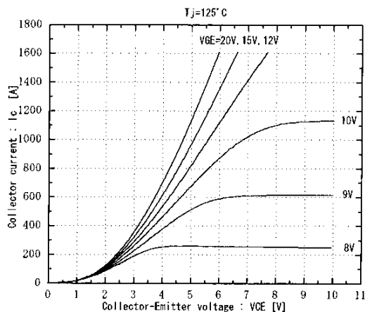
コレクタ電流—コレクタ・エミッタ間電圧特性 Collector current vs. Collector-Emittor voltage (Tj=125°C)
