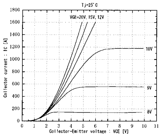
コレクタ電流—コレクタ・エミッタ間電圧特性 Collector current vs. Collector-Emittor voltage (Tj=25°C)
