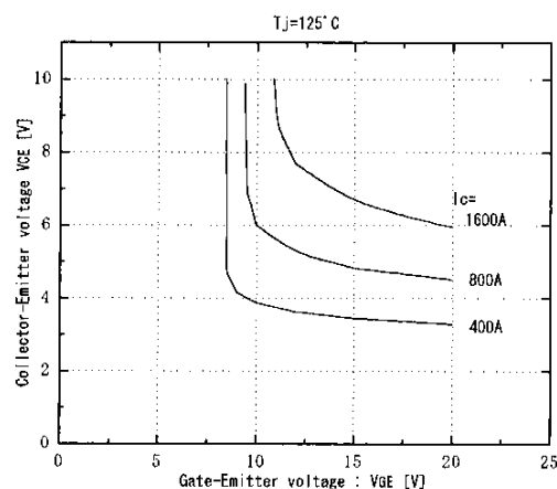
コレクタ・エミッタ間電圧—ゲート・エミッタ間電圧特性 Collector-Emittor voltage vs. Gate-Emittor voltage (Tj=125°C)
