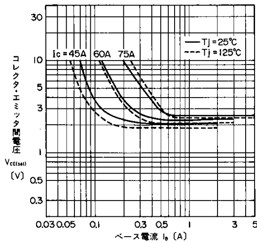
出力特性
