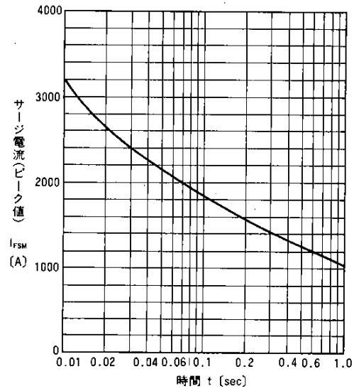
サージ電流 Surge Current
