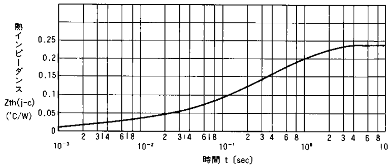
過渡熱インピーダンス(接合-ケース間) Transient Thermal Impedance
