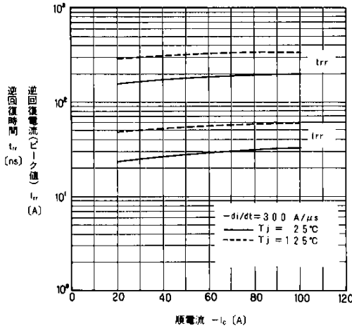
T_{rr} , t_{rr} - I_c 特性 T_{rr} , t_{rr} - I_c
