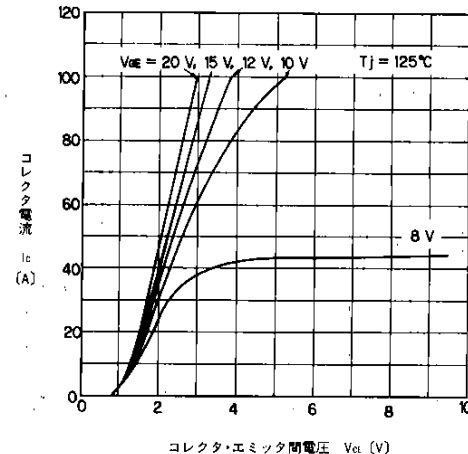
コレクタ電流—コレクタ・エミッタ間電圧特性 Collector Current vs. Collector-Emmitter Voltage
