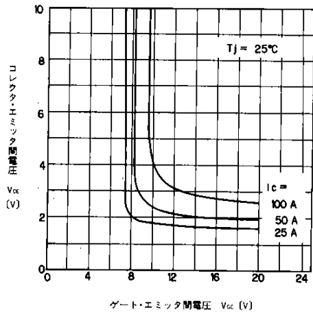
コレクタ・エミッタ間電圧—ゲート・エミッタ間電圧特性 Collector-Emmitter Voltage vs. Gate-Emmitter Voltage
