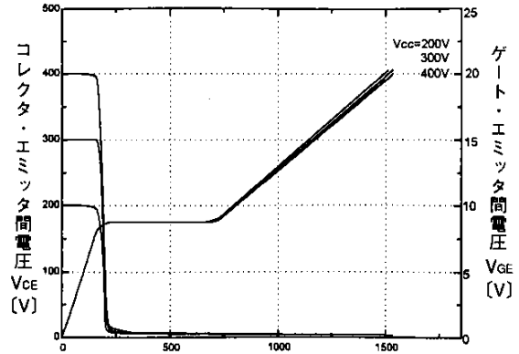
充電電荷量 Q_g [nC] ダイナミック入力特性 ( T_j=25^\circ\text{C} ) Dynamic input characteristic
