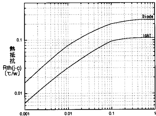
ハルス幅 P_w [S] 過度熱抵抗特性 Transient thermal resistance
