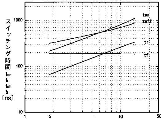
ゲート抵抗 R_g [ \Omega ] スイッチング時間-ゲート抵抗特性 ( T_j=25^\circ\text{C} ) Switching time vs. Gate resistance
