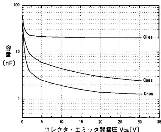
コレクタ・エミッタ間電圧 V_{CE} [V] 容量-コレクタ・エミッタ間電圧特性 ( T_j=25^\circ\text{C} ) Capacitance vs. Collector-Emitter voltage
