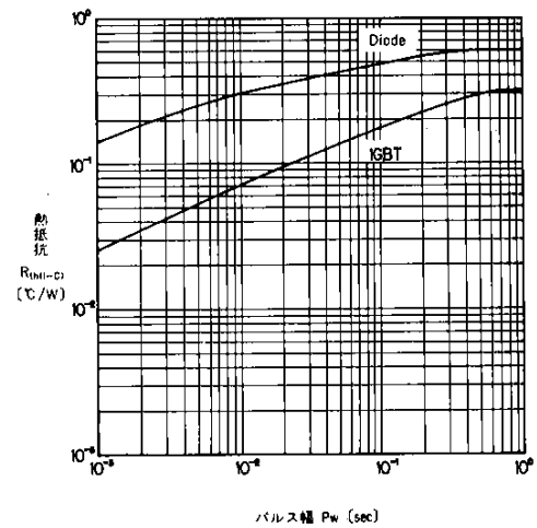
過渡熱抵抗特性 Transient Thermal Resistance
