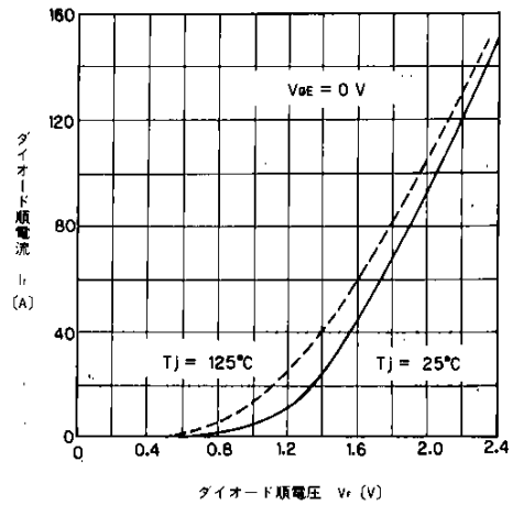
ダイオード順電流 I_f (A) ダイオード順電圧 V_{fr} (V) 高速フリーホイールダイオード順電圧特性 Forward Voltage of Free Wheel Diode
