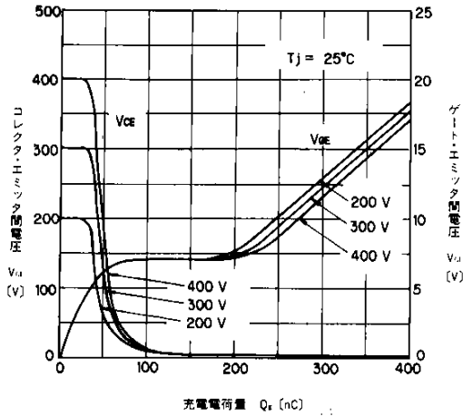
充電電荷量 Q_c (nC) ダイナミック入力特性 Dynamic Input Characteristic
