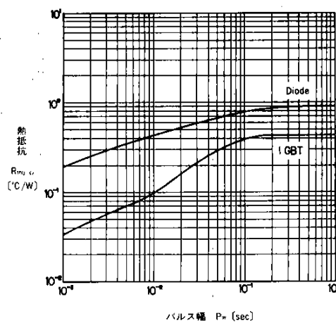
パルス幅 P_w (sec) 過渡熱抵抗 Transient Thermal Resistance
