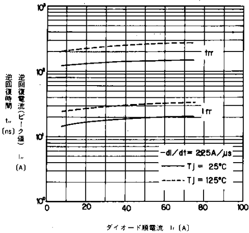
ダイオード順電流 I_f (A) t_{rr} , I_{rr} - I_f 特性 T_{rr} , I_{rr} - I_f
