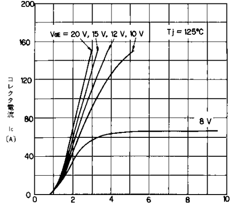
コレクタ・エミッタ間電圧 V_{ce} (V) コレクタ電流—コレクタ・エミッタ間電圧特性 Collector Current vs. Collector-Emitter Voltage
