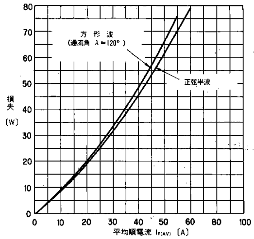
平均順電流特性 - 損失 Output Current vs. Power Loss
