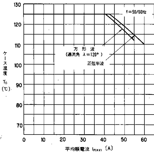
平均順電流 - ケース温度 Average Forward Current vs. Case Temperature
