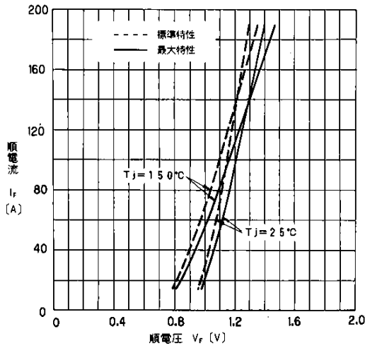
順電圧特性 (1素子あたり) Forward Characteristics
